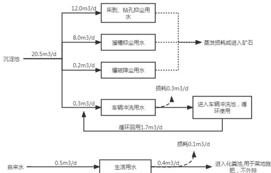
图 4-1 项目水平衡图
