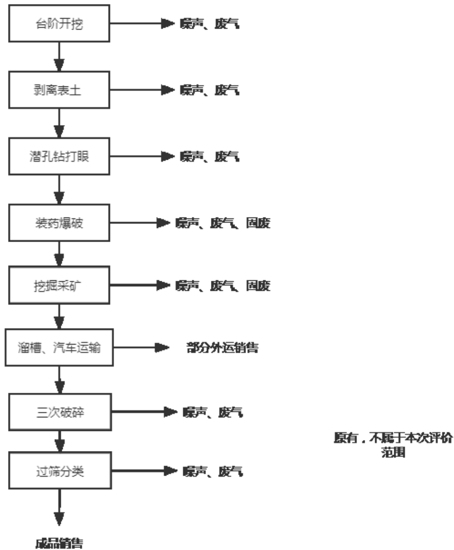
图 4-1 项目生产工艺流程图
